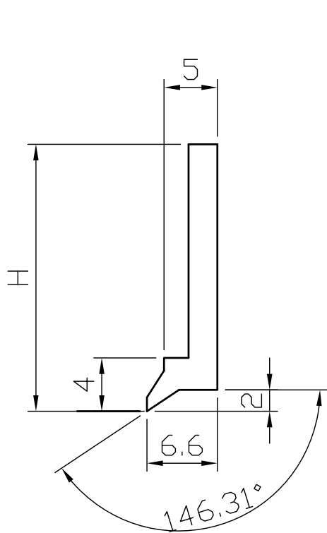
Black rubber(NBR) dimensions
